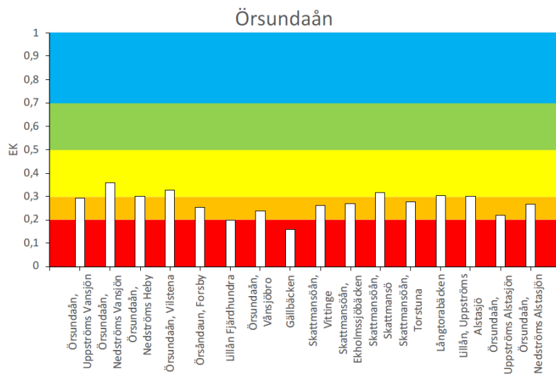
Figur 3. Statusklassning för lokaler i Örsundaåns åtgärdsområde. Blå färg visar hög status, grön färg god status, gul färg måttlig status, orange färg otillfredsställande status och röd färg dålig status.
