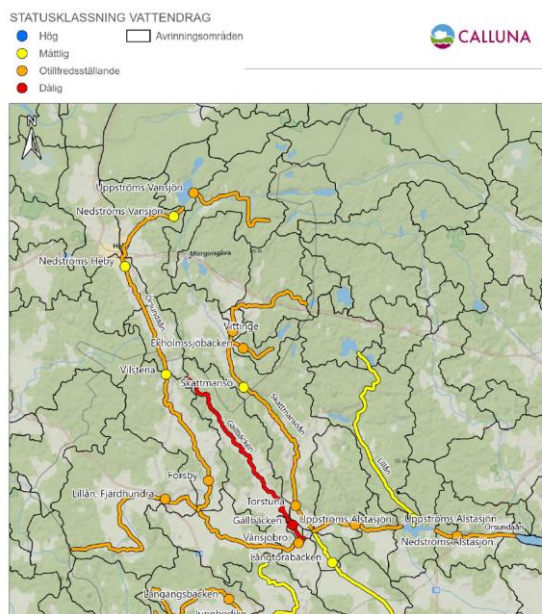
Figur 3. Statusklassning för lokaler i Örsundaåns åtgärdsområde. Blå färg visar hög status, grön färg god status, gul färg måttlig status, orange färg otillfredsställande status och röd färg dålig status.
