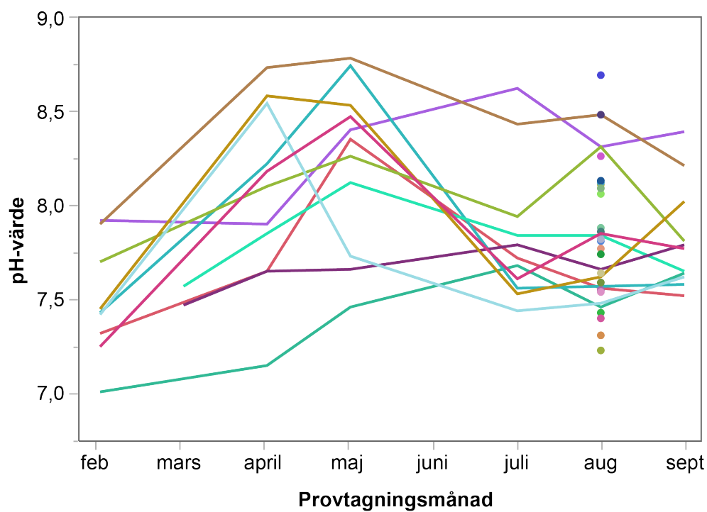
Figur 16. Variationen i ytvattnets pH-värde i Mälaren under 2017. Färgkoderna för de olika provplatserna ges i tabell 6. Provplatser som endast provtogs i augusti illustreras med punkter.
