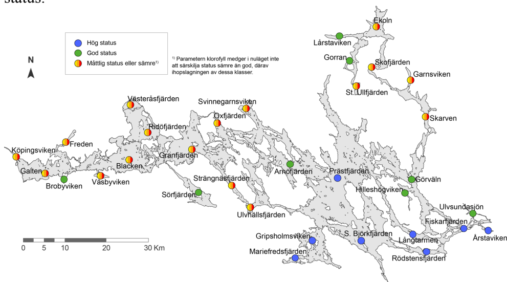
Figur 19. Statusklassning av klorofyll a i Mälarens ytvatten i augusti 2017. OBS! Endast resultat från ett enda tillfälle har använts för att kunna jämföra de olika provplatserna. Referensvärdena har hämtats från VISS.
