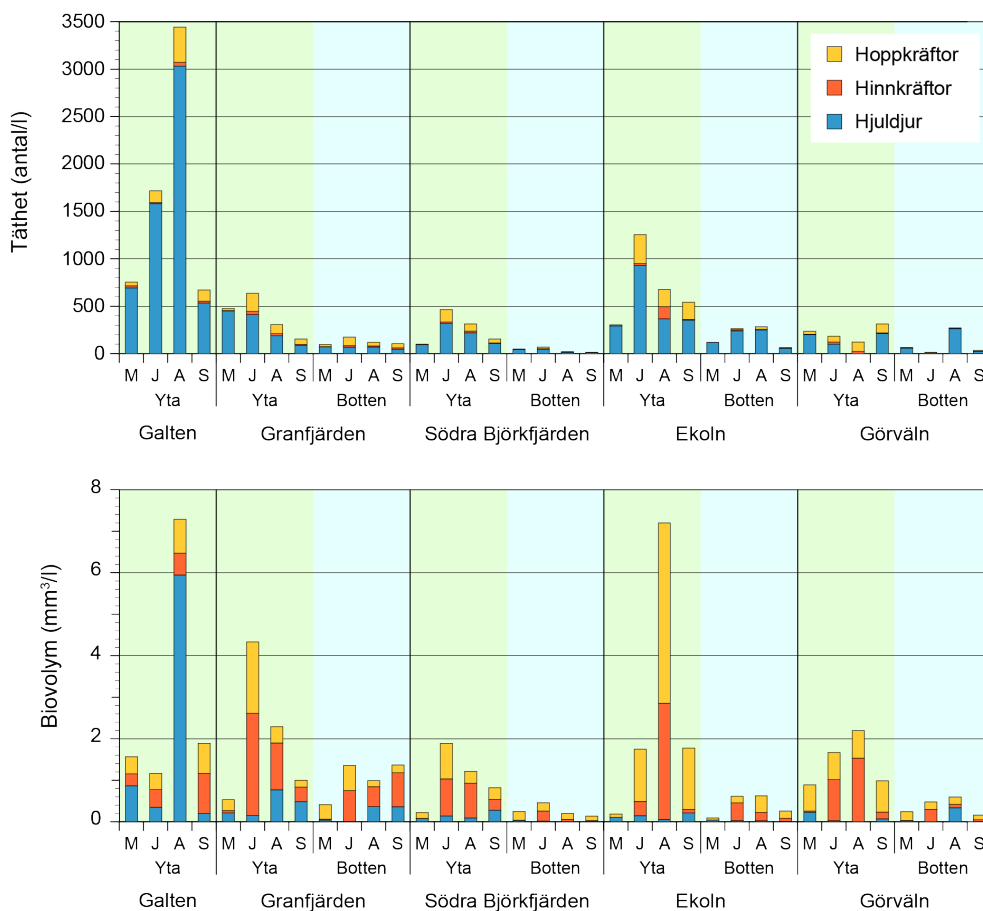
Figur 23. Tätheter (antal/l) och biovolym (mm 3 /l) av de tre stora djurplanktongrupperna i Mälaren i maj, juli, augusti och september 2017. Prover togs i ett ytligt vattenskiert 0–10 samt om möjligt i ett djupare skikt från 15 m ned till 25–40 m beroende på provplatsens vattendjup. I Galten tas endast i det ytligare skiktet på grund av det ringa vattendjupet.
