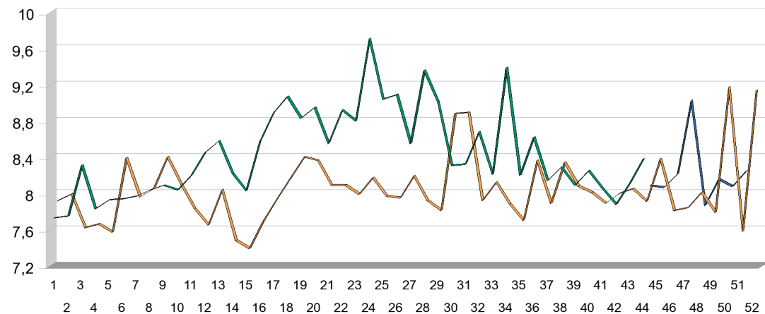
TOC, mg/l
