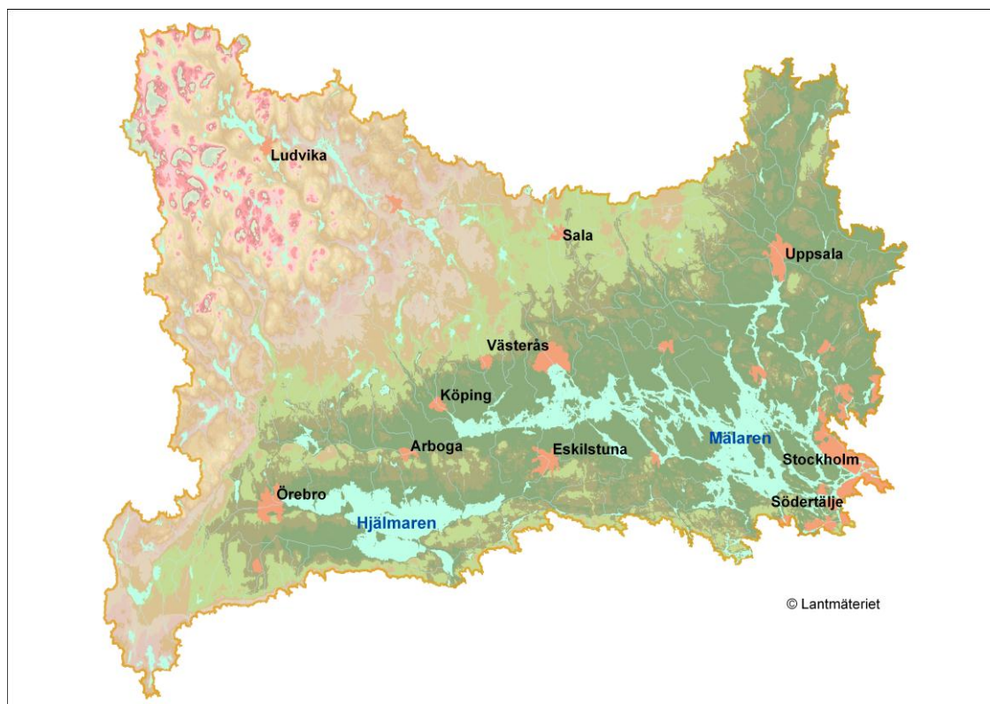
Figur 2. Mälarens avrinningsområde.
